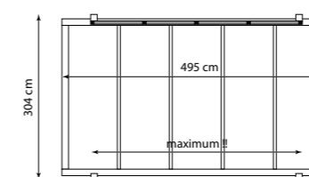
4 wand-elementen + 3 palen
