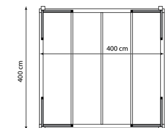
8 wand-elementen + 8 palen
